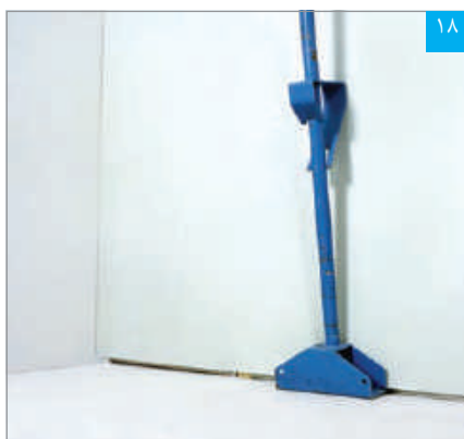
۱۸ پنل‌ها بوسیله جک مخصوص به نحوی بر روی زیرسازی قرار می‌گیرند که ۱ سانتی‌متر با کف فاصله داشته باشند
