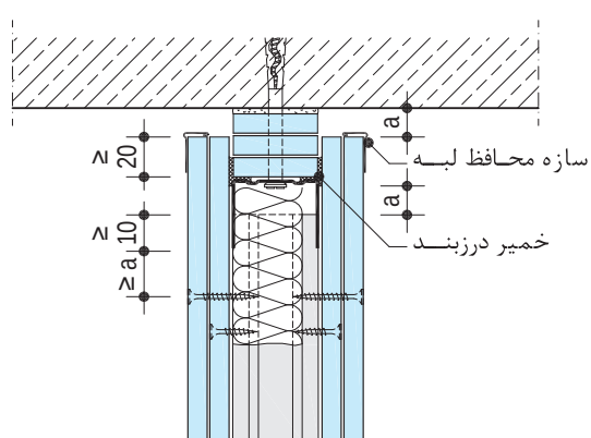
اتصال دیوار به سقف کاذب (برای سقف کاذب دارای کد حریق از بالا یا از پایین و بالا)
