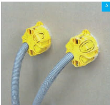
گیره‌ها با پنل درگیر شده و قوطی برق در جای خود محکم می‌شود
