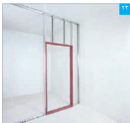
۲۳ قاب بندی و تقویت بازشوی در تکمیل شده
