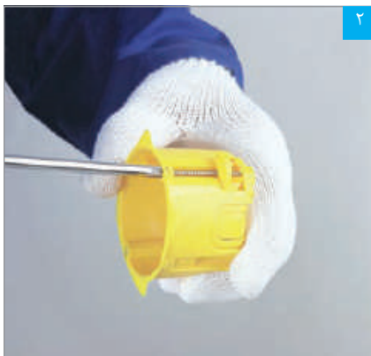
گیره‌های متحرک قوطی برق توسط پیچ گوشتی قابل تنظیم می‌باشند
