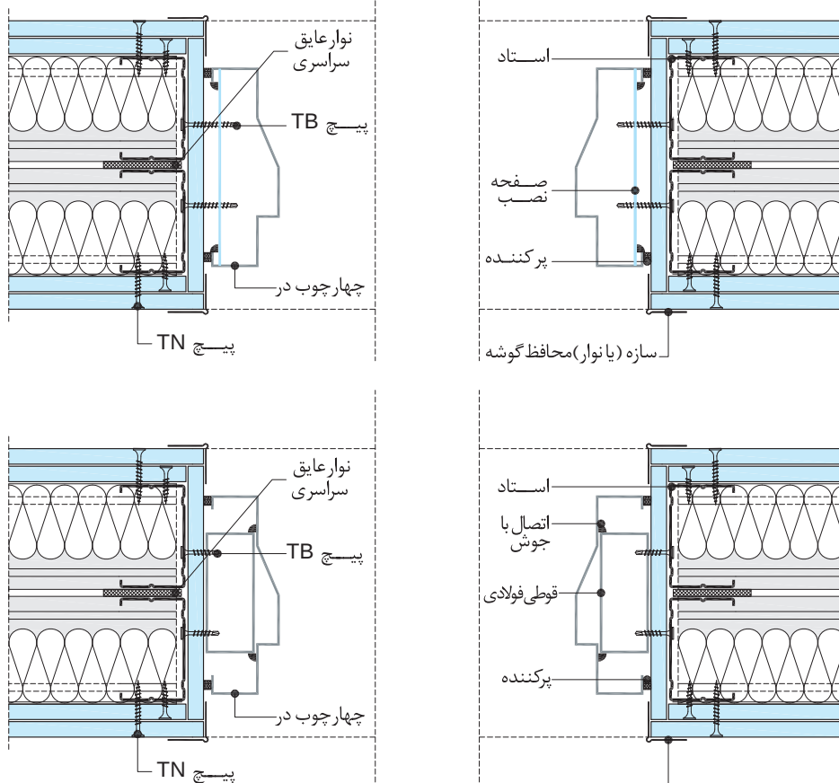
جزئیات نصب چهارچوب در (W115.ir)
