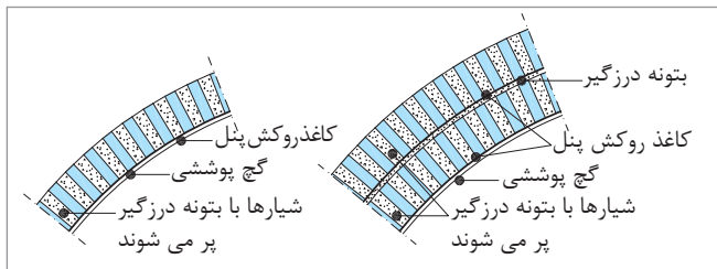
پوشش کاری دو لایه و تک لایه
