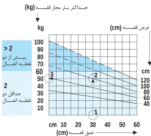
نمودار ۱: بارگذاری دیوارهای W111.ir و W115.ir
