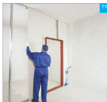
اجرای پنل دوم دور چهارچوب
