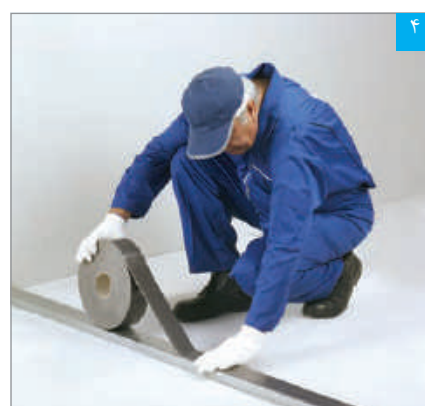
۴ اجرای نوار عایق (یا دو ردیف خمیر سیلیکون) بر پشت جان رانر کف و سقف
