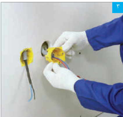
در حالی که گیره‌ها باز هستند، قوطی برق در محل خود قرار می‌گیرد
