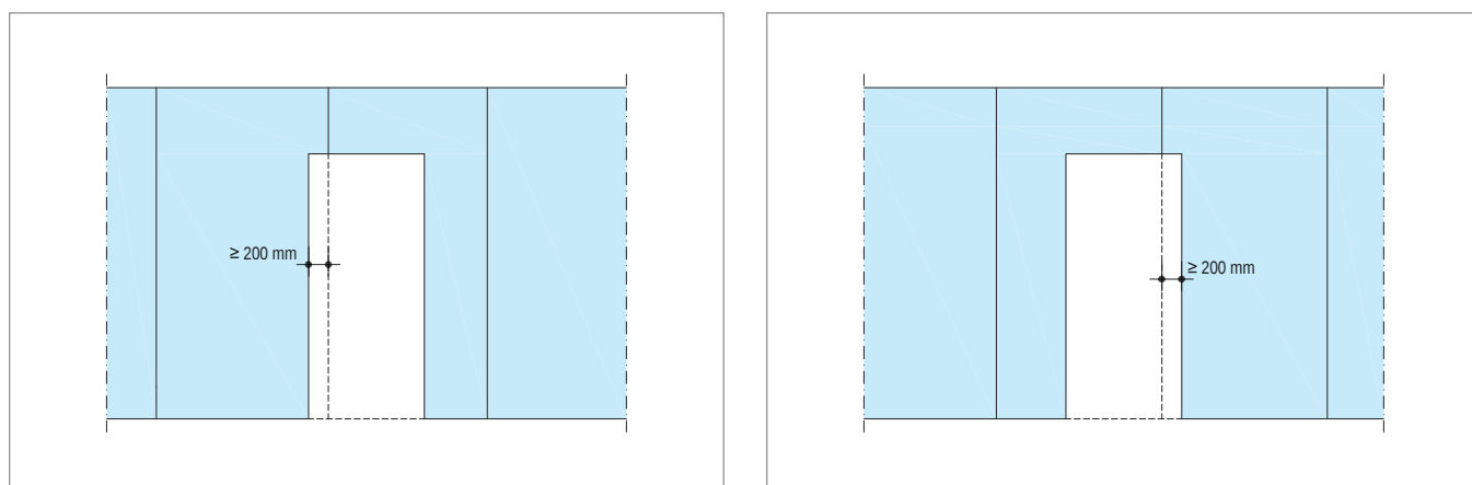
پوشش‌کاری سمت دوم (به اصول حصیرچینی پنل‌ها در دو سمت دیوار توجه شود)
