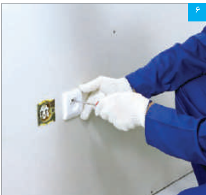
پس از نصب قوطی، پرز برق نصب می‌شود
